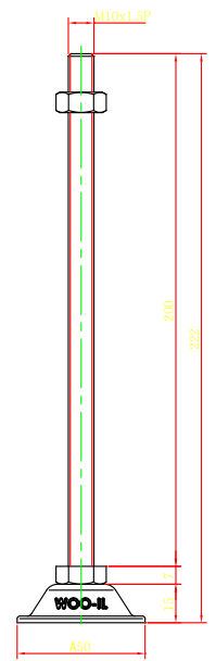
BL50-M10-200
