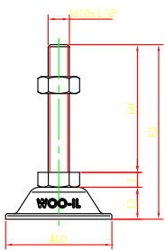
BL50-M10-60
