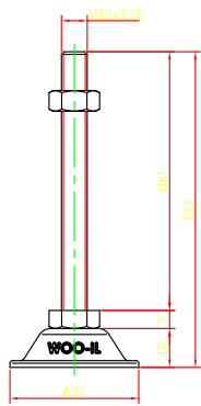
BL50-M10-100
