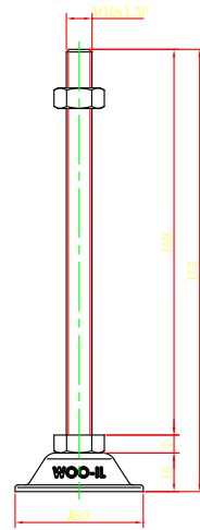
BL50-M10-150
