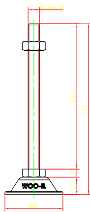
BL50-M10-125
